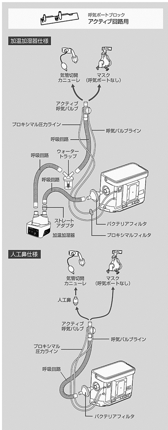
図2 シングルブランチ回路例 (トリロジー100 plus ® フィリップス社製) トリロジー100plus簡易取扱説明書より
