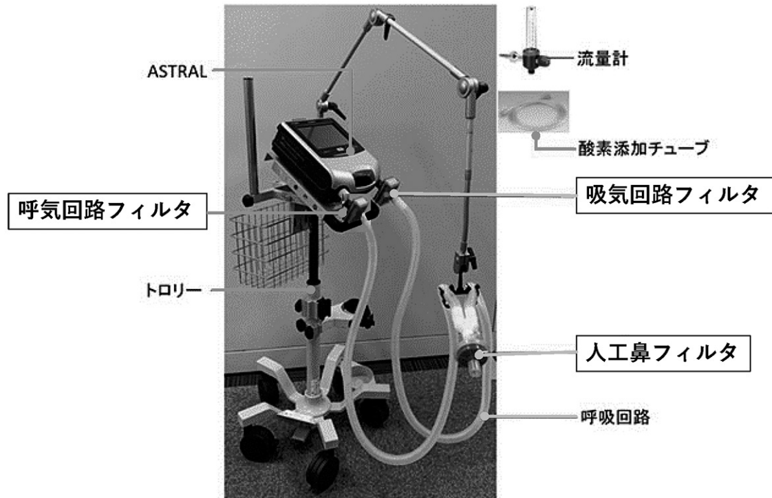
図3 ダブルブランチ回路例 (クリーンエアASTRAL150® ResMed社製)
